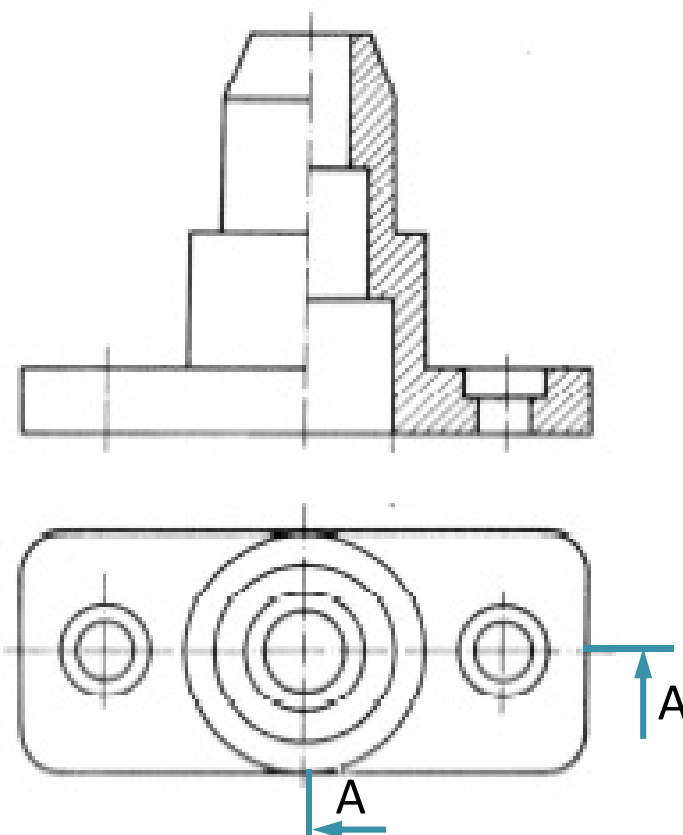
Presjek A-A
