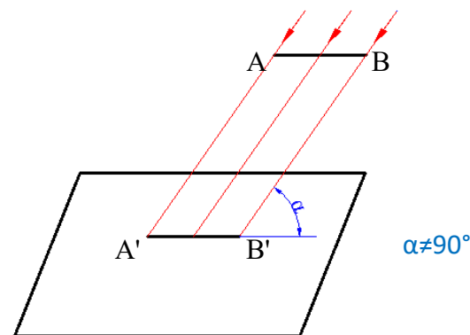
Kosa (kosougla) projekcija
