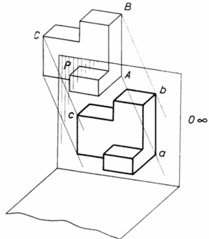
Koso projiciranje
